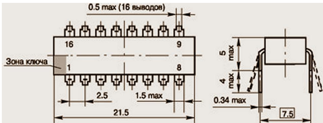
Микросхема КР590КН5
