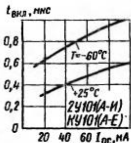
Зависимости времени включения от тока
