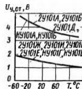
Зависимости отпирающего постоянного напряжения управления от температуры
