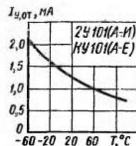
Зависимость отпирающего постоянного тока управления от температуры
