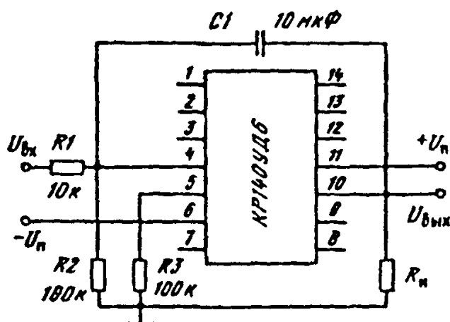
Типовая схема включения КР140УД6
