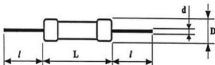
Габаритные размеры резисторов С2-10:
