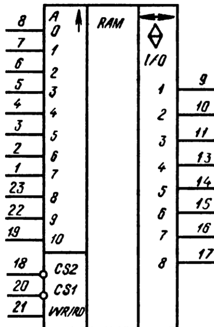
Условное графическое обозначение К537РУ8, КН537РУ8, КР537РУ8
