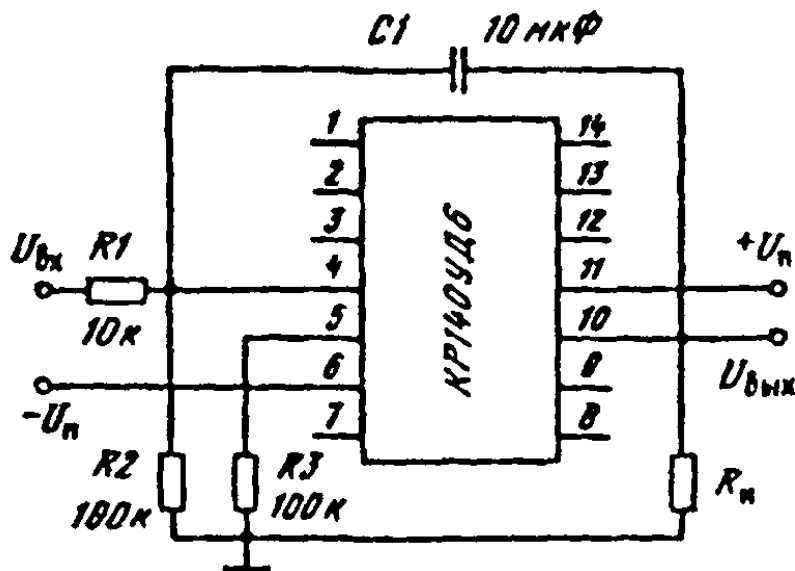
Типовая схема включения КР140УД6
