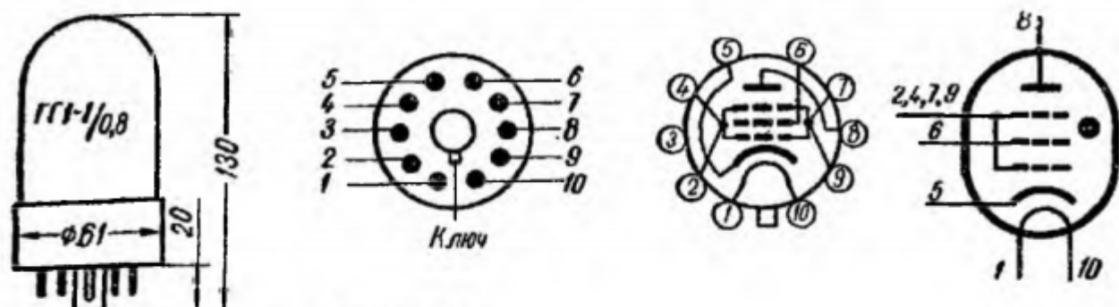
Рис. 28. Тиратрон ТГ1-1/0,8:
