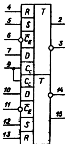
Условное графическое обозначение К700ТМ131-2
