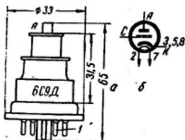
Рис. 484. Лампа 6С9Д:
