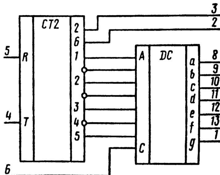
Условное графическое обозначение К176ИЕЗ
