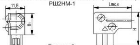
Рисунок 3 Вилка в прямом металлическом кожухе или в прямом пластмассовом кожухе РШ2Н-1, РШ2НП-1
