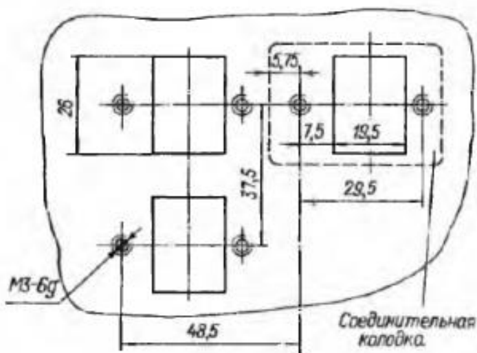
Рис. 2-119. Разметка для крепления
