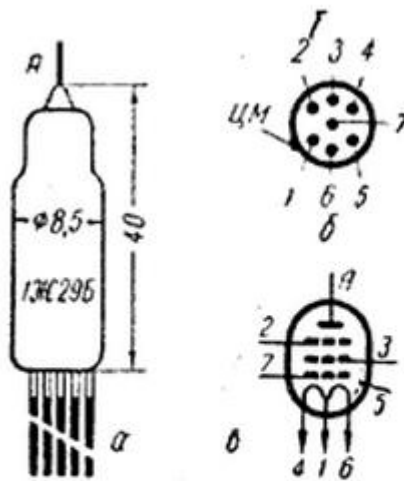
Рис. 47. Лампа 1Ж29Б:
