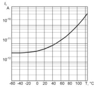
Типовая зависимость входного тока от температуры среды
