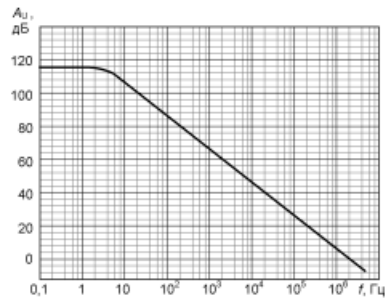
Типовая зависимость коэффициента усиления от частоты
