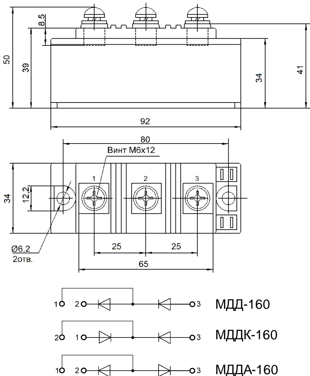
Рис. 11. Габаритные и установочные размеры
