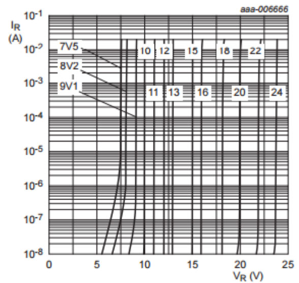
BZX84-A/B/C7V5 to BZX84-A/B/C24 T_{amb} = 25\text{ }^\circ\text{C}
