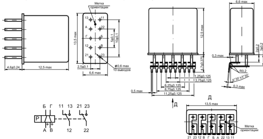
Рис. 1 - Общий вид реле РПС45 исполнения РС4.520.755, -01 ... -10; РС4.520.756, -01 ... -10, -21 и принципиальная электрическая схема
