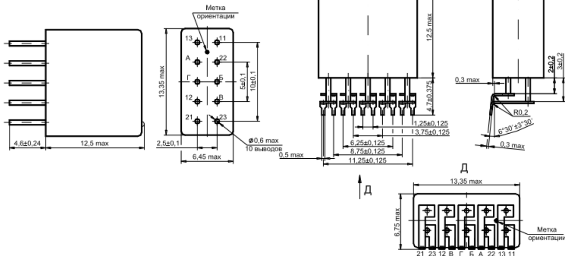
Рис. 3 - Общий вид реле РПС45 исполнения РС4.520.755-30 ... -35; РС4.520.756-30 ... -35
