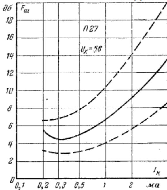
Зависимость коэффициента шума от тока коллектора*
