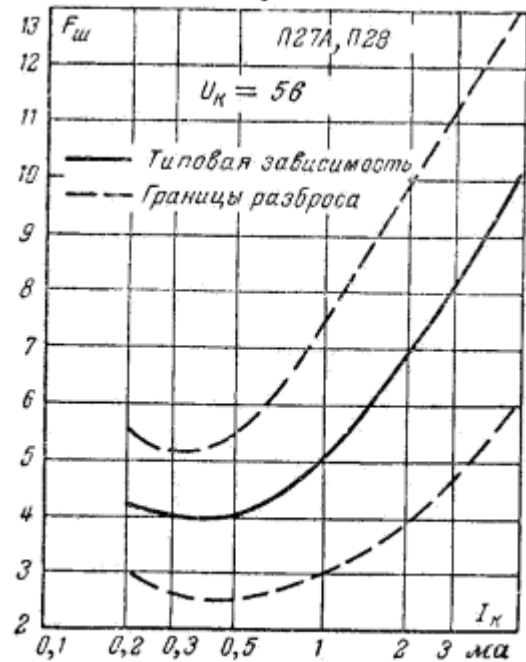
Зависимость коэффициента шума от тока коллектора*
