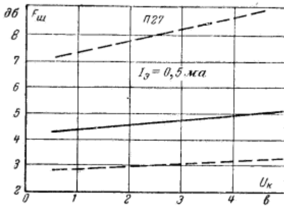
Зависимость коэффициента шума от напряжения коллектора*
