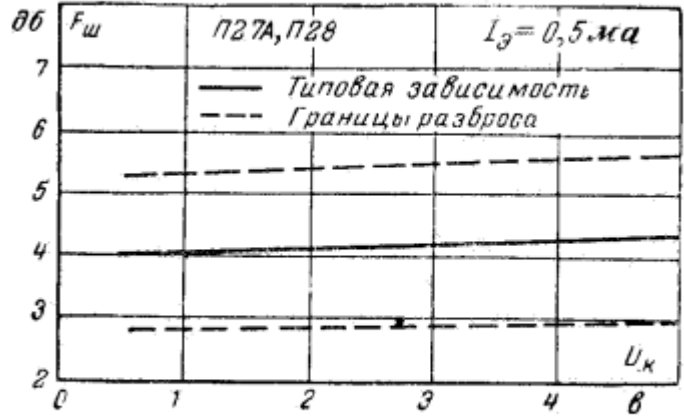
Зависимость коэффициента шума от напряжения коллектора*
