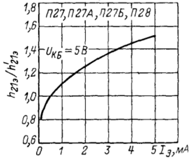
Зависимость относительного коэффициента передачи тока в режиме малого сигнала от напряжения коллектор-база от тока эмиттера
