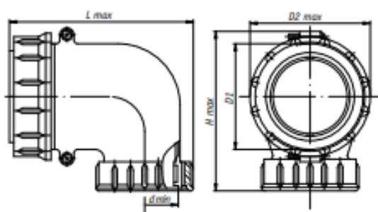
Рисунок 8 - Вилки и розетки типов ШР и СШР кабельные с угловым патрубком и гайкой для экранированного кабеля
