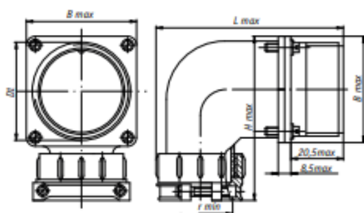
Рисунок 5 - Вилки и розетки типа ШР приборные с угловым патрубком и гайкой для неэкранированного кабеля
