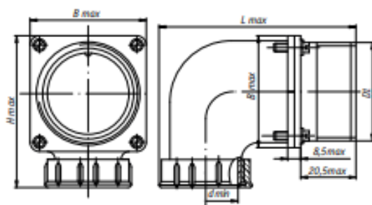
Рисунок 4 - Вилки и розетки типа ШР приборные с угловым патрубком и гайкой для экранированного кабеля
