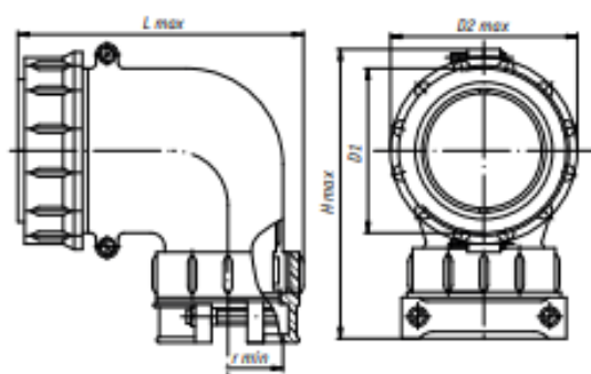
Рисунок 9 - Вилки и розетки типа ШР кабельные с угловым патрубком и гайкой для неэкранированного кабеля
