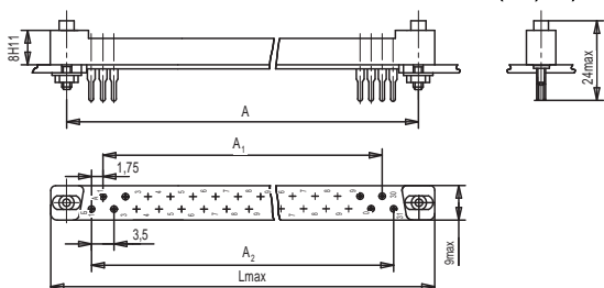
Вилка ГРПМШ-1-31(45,61)ГП2
