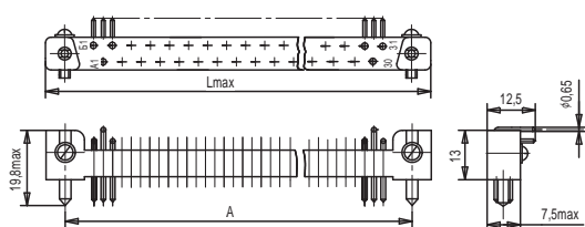
Вилка ГРПМШ-1-31(45,61)ШУ2
