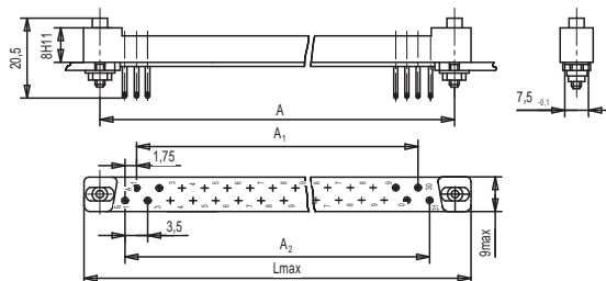
Вилка ГРПМШ-1-31(45,61)ГО2
