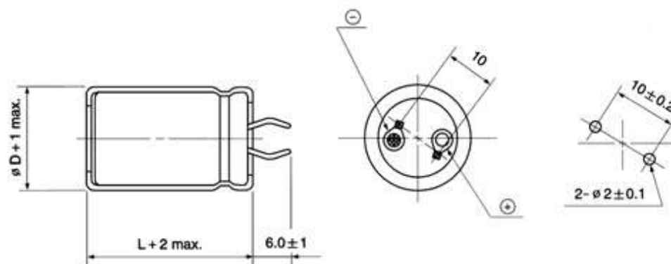
Размеры сетевых конденсаторов ELZET CD294
