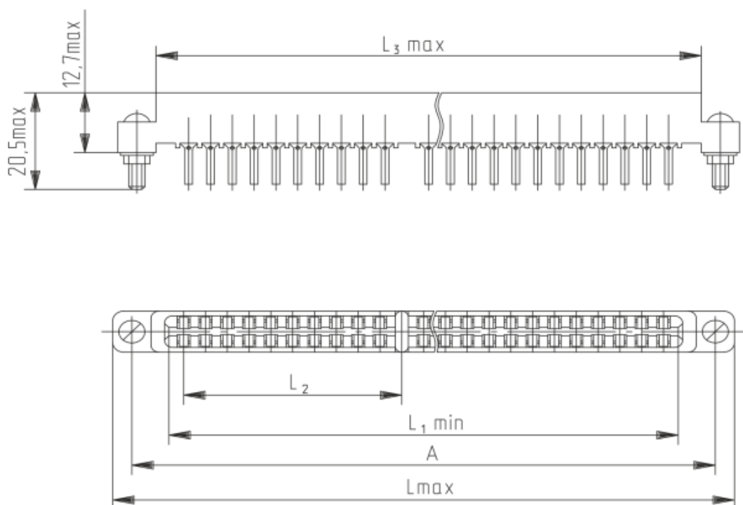
Рисунок 1 Соединители (розетки) типа РГ1Н-3
