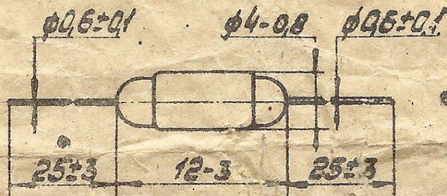
Габаритный чертеж
