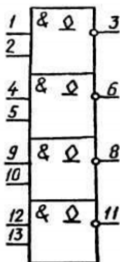
Условное графическое обозначение КР1533ЛА9, КФ1533ЛА9, ЭКА1533ЛА9, ЭКФ1533ЛА9
