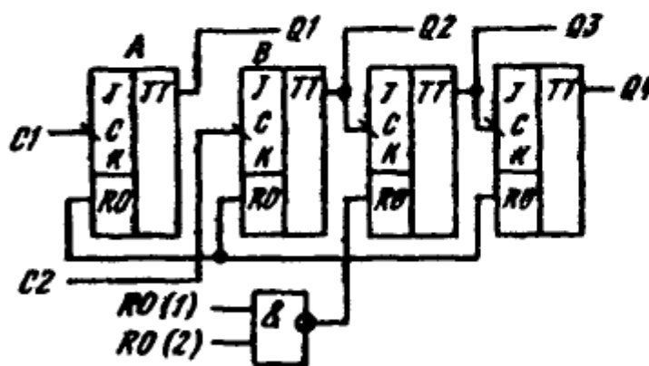
Функциональная схема K155IE5, KM155IE5
