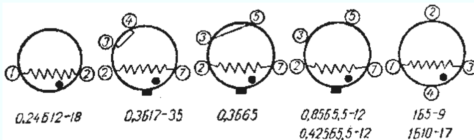
Электрические данные бареттеров
