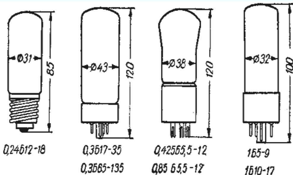
Основные размеры бареттеров
