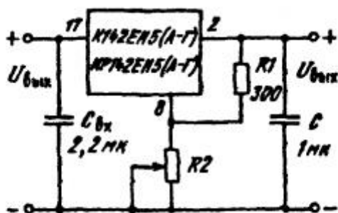
Схема включения K142EH5 (А — Г), KP142EH5 (А — Г) на повышенные значения выходного напряжения
